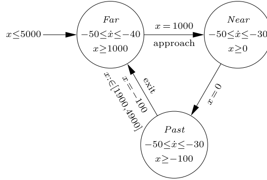
Fig. 8. Train automaton.
