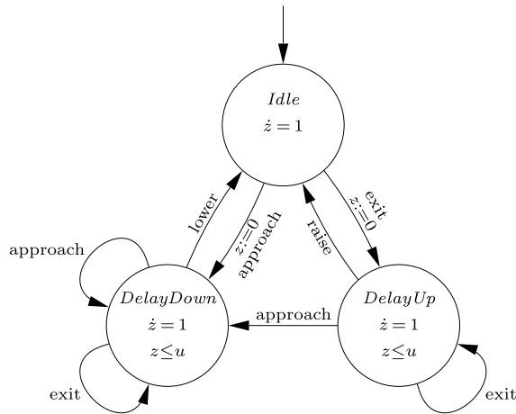
Fig. 10. Controller automaton.
