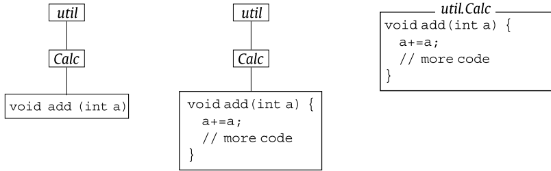
Fig. 3. FST, FST equipped with code, and compressed FST.
